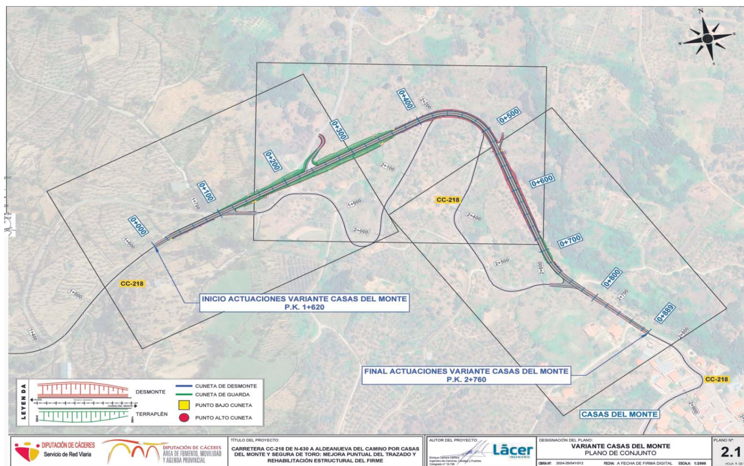
Plano de la actuación de la variante que se proyecta para eliminar una serie de curvas peligrosas.
